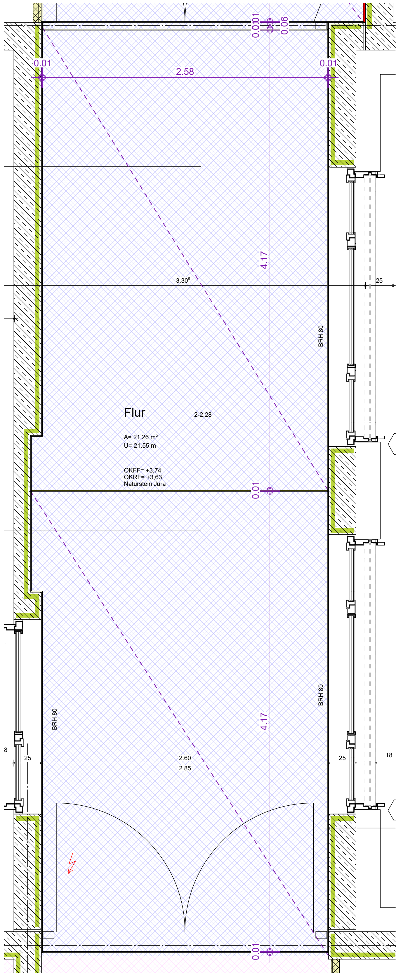
OG GRUNDRISSAUSSCHNITT ESTRICHARBEITEN FLUR 2-2.28 M 1:20
