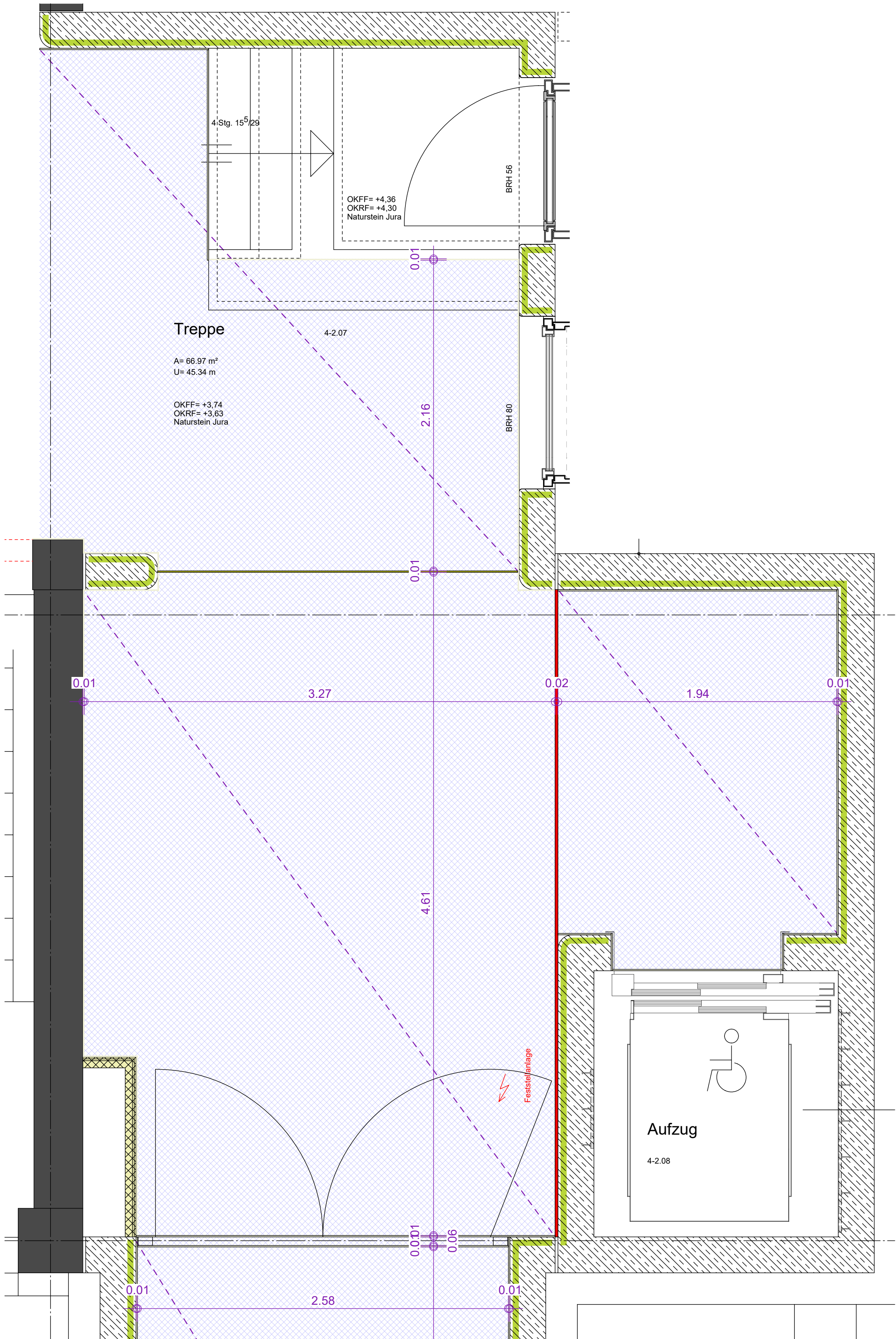
OG GRUNDRISSAUSSCHNITT ESTRICHARBEITEN TREPPE 4-2.07 M 1:20
